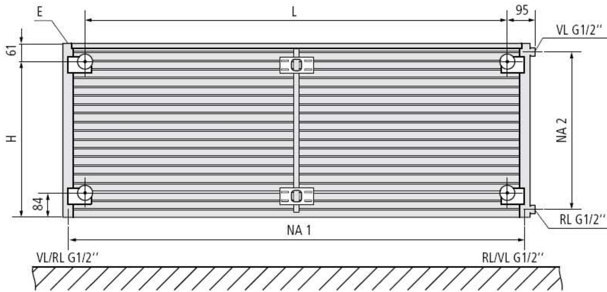
Vorderansicht
