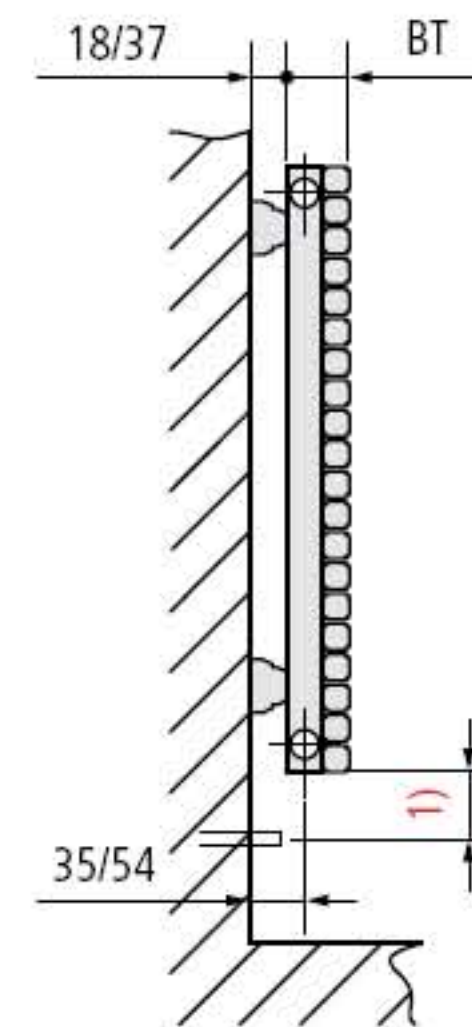
Seitenansicht
