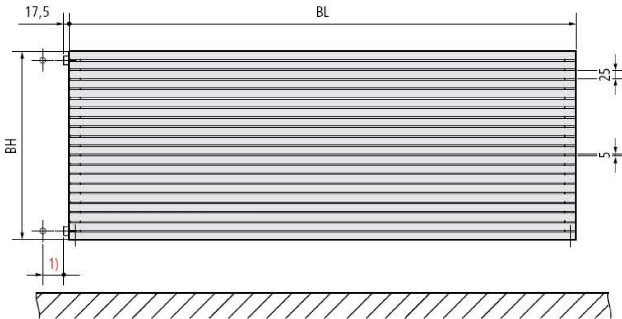
Vorderansicht
