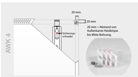
Winkel werden beidseitig (oberhalb vom Heizkörper) an der Wand befestigt.
